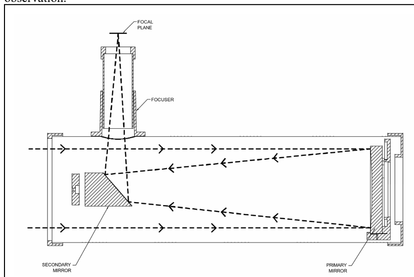
Figur 3-2 Genomsnitt av ljusbanan för Newton-refraktorns optiska design
