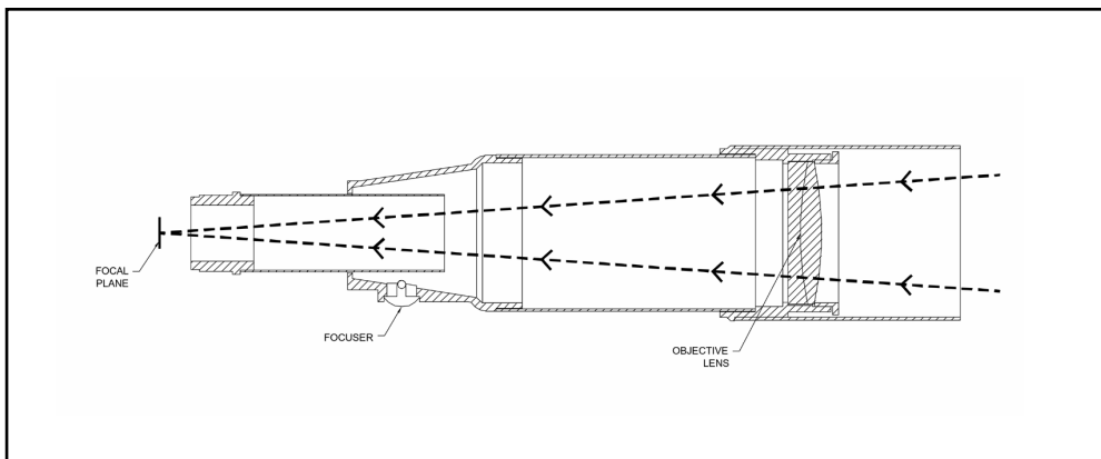
Figur 3-1 Genomsnitt av ljusbanan för refraktorns optiska design
